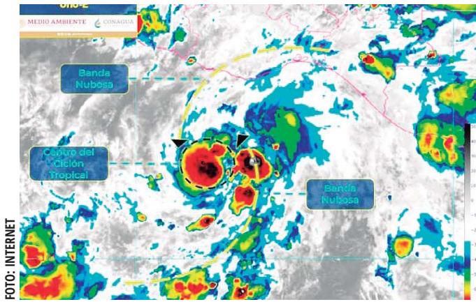
La Depresión Tropical Uno-E daría origen al huracán Ágatha.
