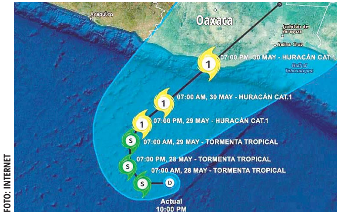
Como huracán categoría 1, impactaría en las costas de Oaxaca.
